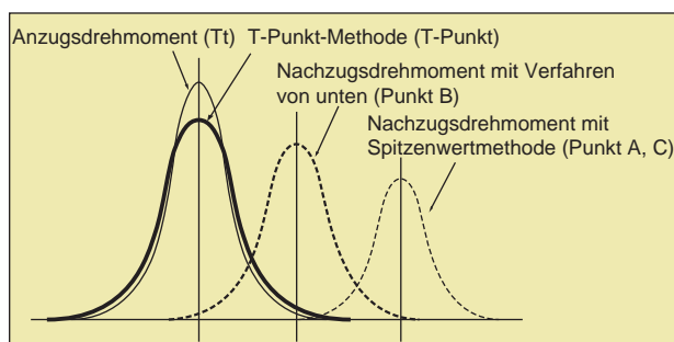
Abbildung-3 Verteilung-Nachzugsdrehmoment
